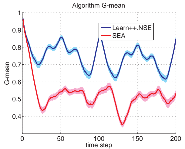
(j) G-mean
