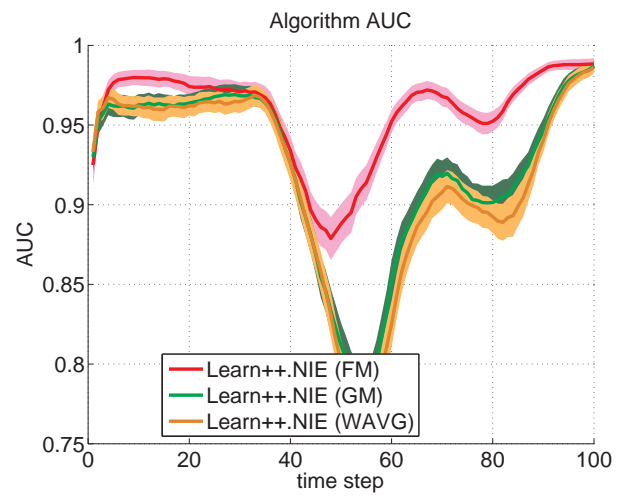
(b) AUC
