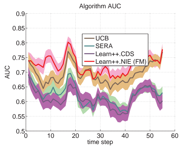
(b) AUC
