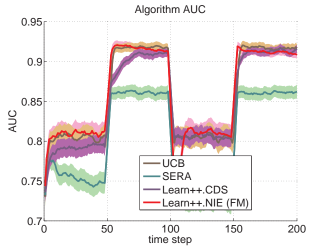
(b) AUC
