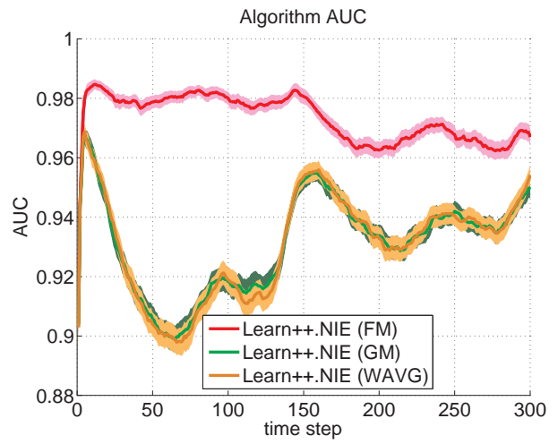
(b) AUC
