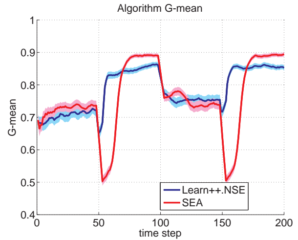
(d) G-mean
