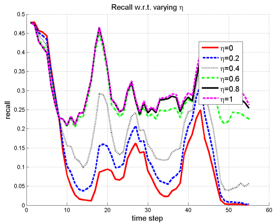
(d) Recall
