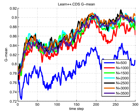
(d) G-mean
