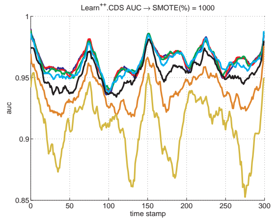
(d) SMOTE(%)=1000
