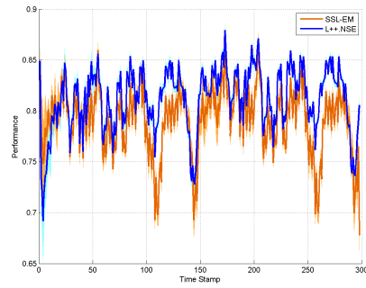
(b) Bias=1
