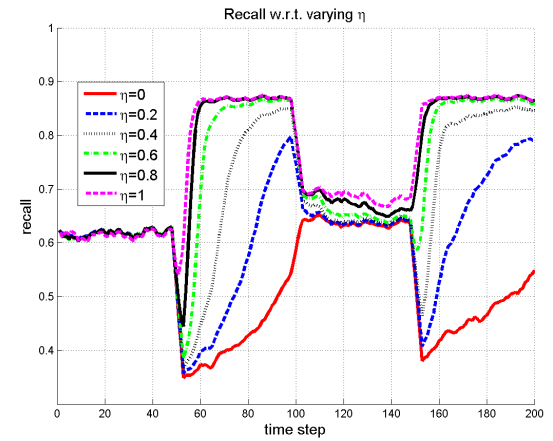
(d) Recall
