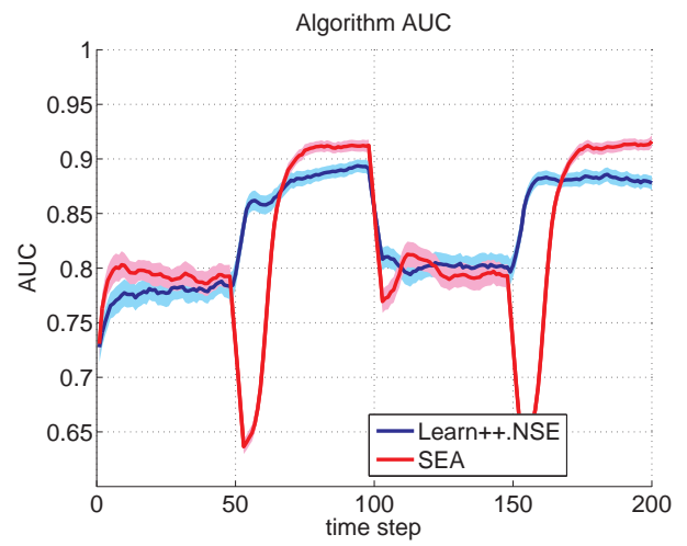
(b) AUC
