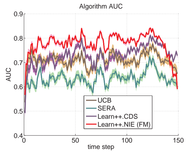
(b) AUC
