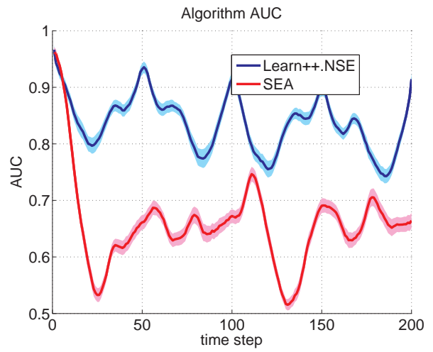
(h) AUC
