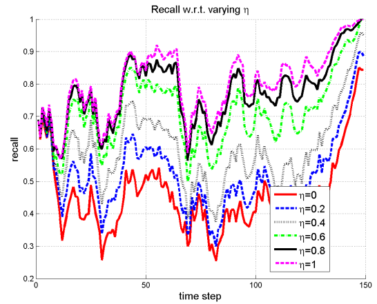
(d) Recall
