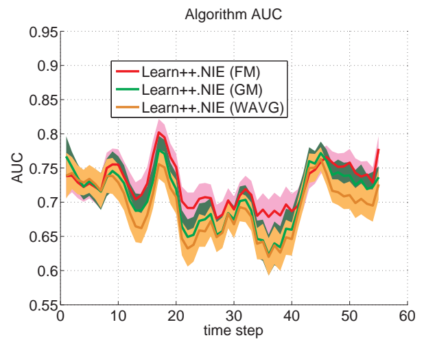
(b) AUC
