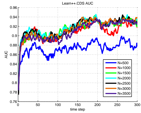
(b) AUC
