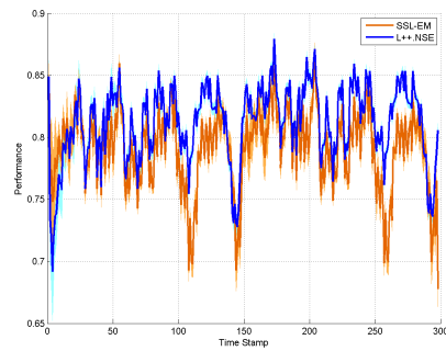
(d) Bias=5
