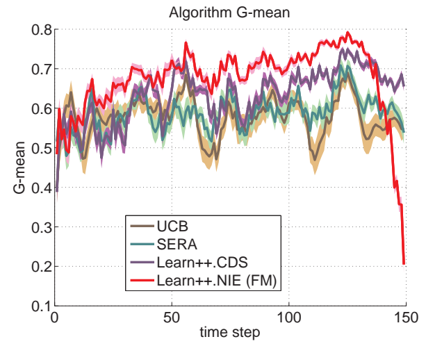
(d) G-mean
