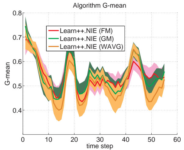
(d) G-mean
