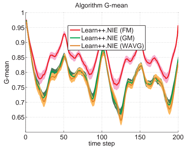
(d) G-mean
