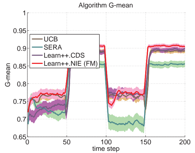
(d) G-mean
