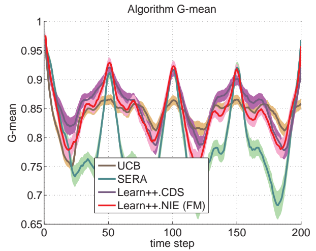
(d) G-mean
