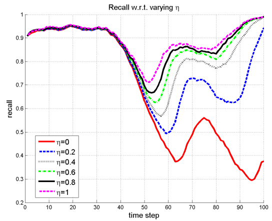
(d) Recall
